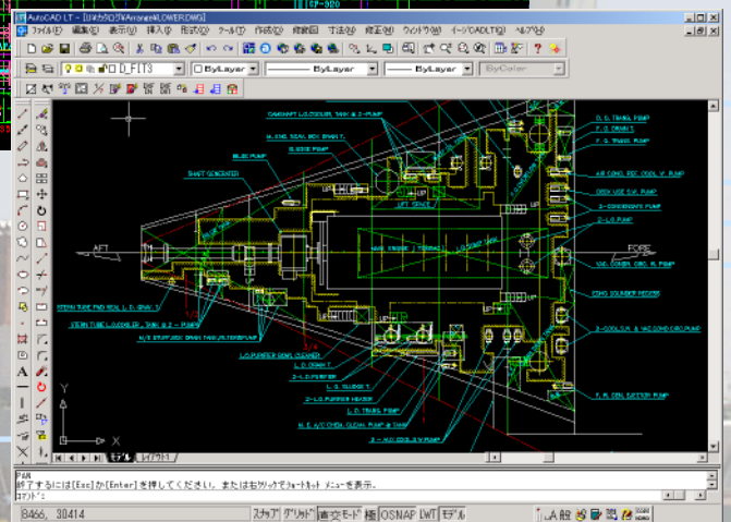
機関室配置図
