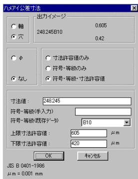
はめあい公差
