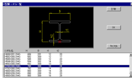
形鋼シンボル
